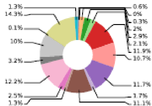
2004 - conta_pazienti
