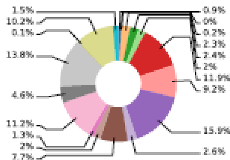
2013 - conta_pazienti
