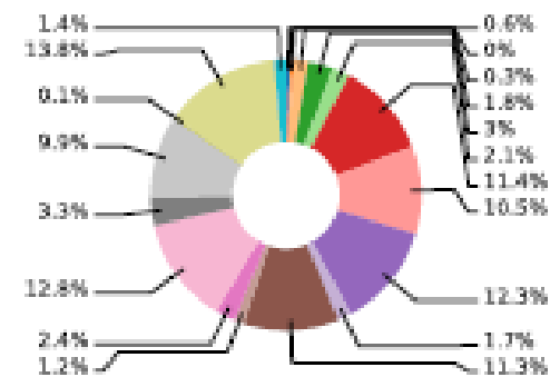
2005 - conta_pazienti
