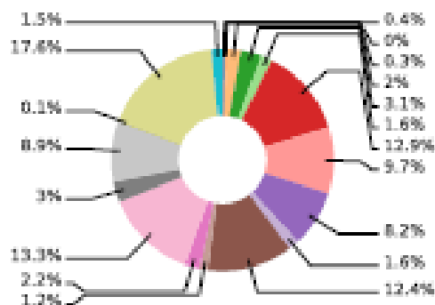
2003 - conta_pazienti
