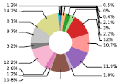
2003 - conta_pazienti
