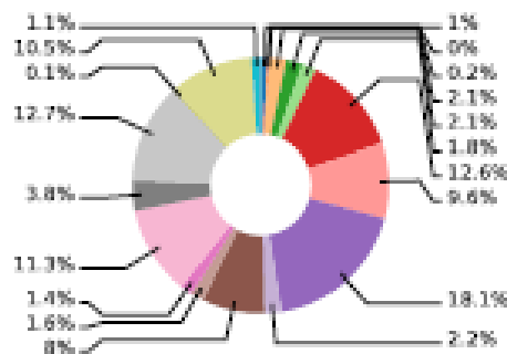
2010 - conta_pazienti
