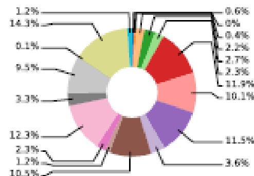
2005 - conta_pazienti
