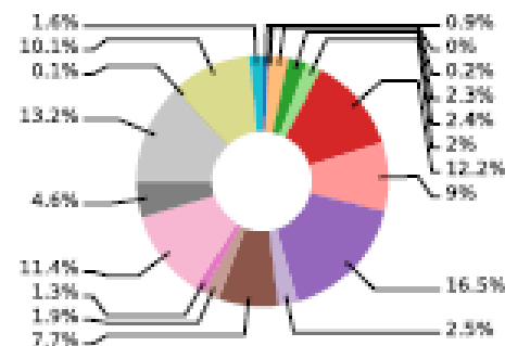
2011 - conta_pazienti
