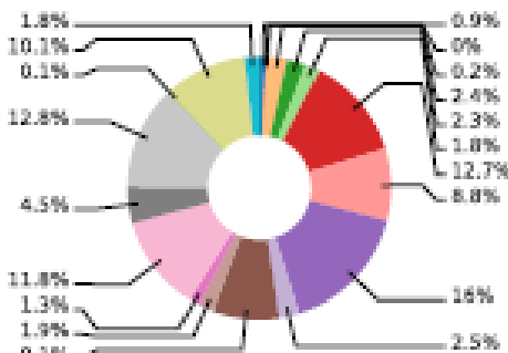
2012 - conta_pazienti
