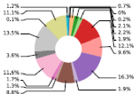
2009 - conta_pazienti
