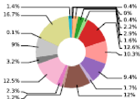
2004 - conta_pazienti
